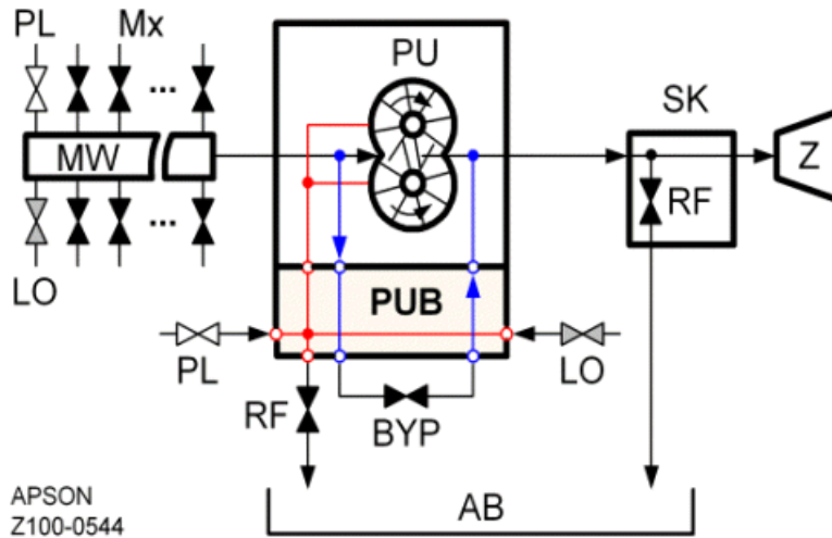
APSON Pumpenspülblock CPY-2000
